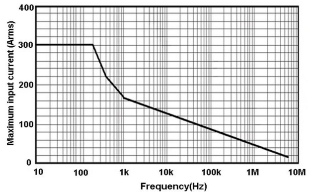
图 11.a HCP8300 最大测量电流 VS 频率曲线 (超过该曲线所示最大电流连续使用会导致探头烧毁)
