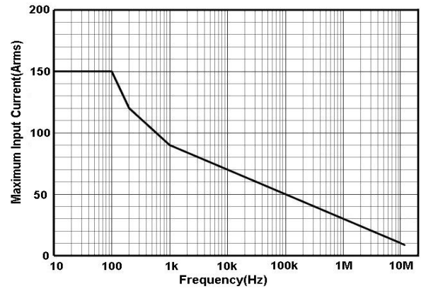
图 8.a HCP8150 最大测量电流 VS 频率曲线
