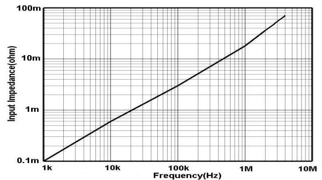
图 15 HCP8500 输入阻抗 VS 频率曲线
