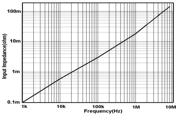
图 12.b HCP8300A 输入阻抗 VS 频率曲线
