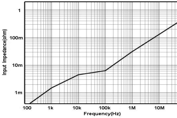
图 6 HCP8050 输入阻抗 VS 频率曲线
