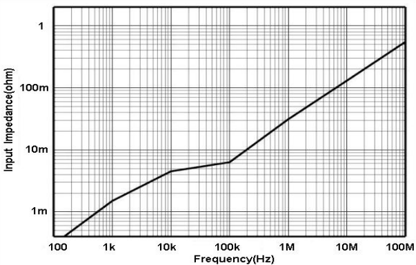
图 3.c HCP8030D 输入阻抗 VS 频率曲线
