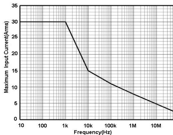
图 2.b HCP8030C 最大测量电流 VS 频率曲线
