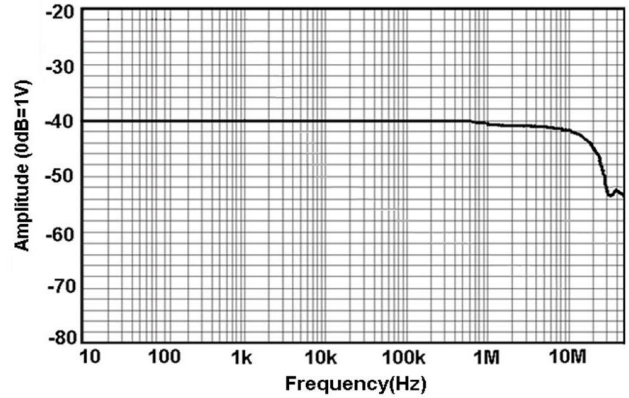
图 7.a HCP8150 幅频曲线
