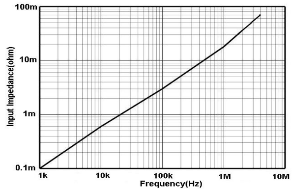
图 12.a HCP8300 输入阻抗 VS 频率曲线
