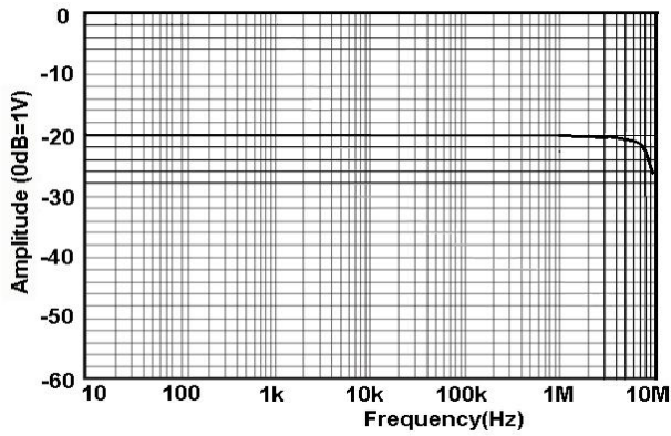
图 10 .b HCP8300A 幅频曲线
