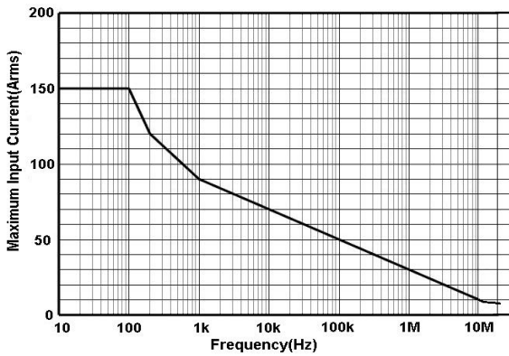
图 8.b HCP8150A 最大测量电流 VS 频率曲线
