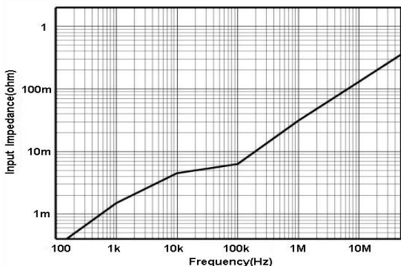
图 3.a HCP8030 输入阻抗 VS 频率曲线
