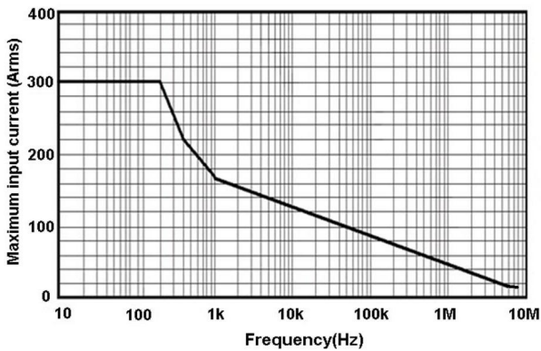
图 11.b HCP8300A 最大测量电流 VS 频率曲线 (超过该曲线所示最大电流连续使用会导致探头烧毁)
