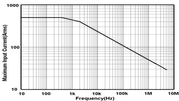
图 14 HCP8500 最大测量电流 VS 频率曲线 (超过该曲线所示最大电流连续使用会导致探头烧毁)
