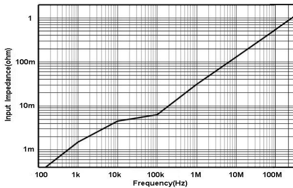
图 3.d HCP8030H 输入阻抗 VS 频率曲线
