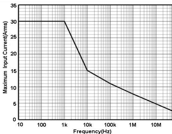
图 2.a HCP8030 最大测量电流 VS 频率曲线
