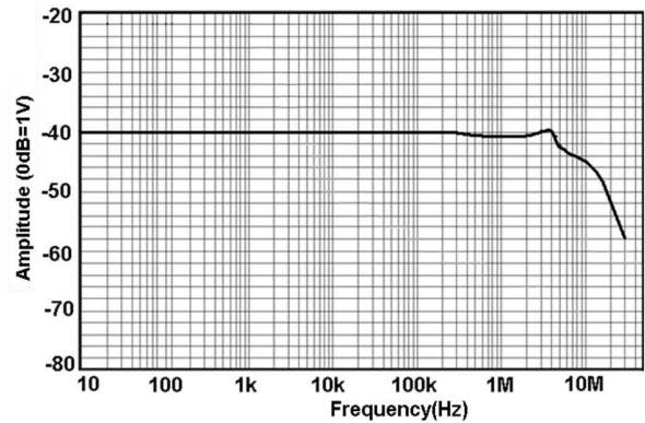
图 13 HCP8500 幅频曲线
