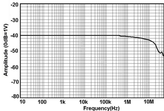
图 10.a HCP8300 幅频曲线
