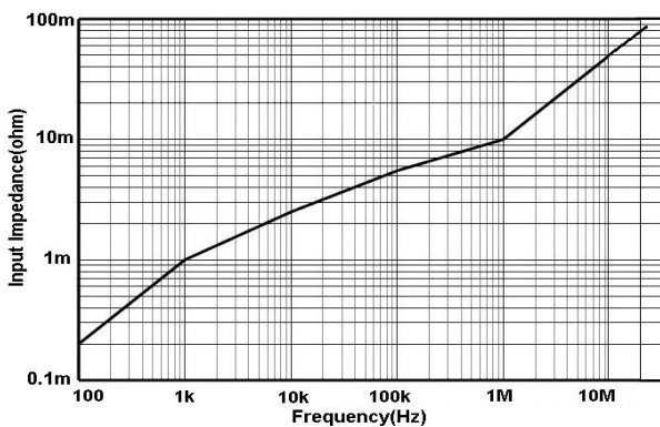
图 9.b HCP8150A 输入阻抗 VS 频率曲线
