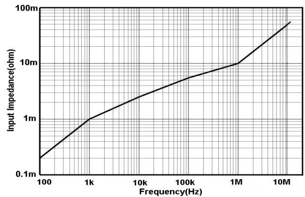
图 9.a HCP8150 输入阻抗 VS 频率曲线
