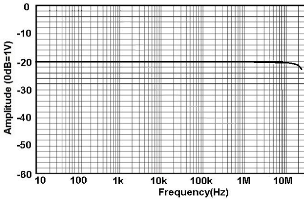
图 7.b HCP8150A 幅频曲线
