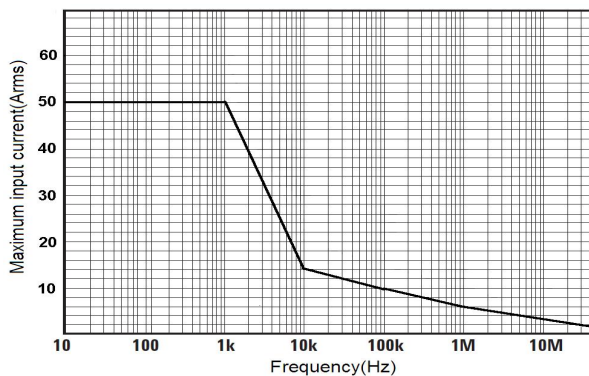
图 5 HCP8050 最大测量电流 VS 频率曲线
