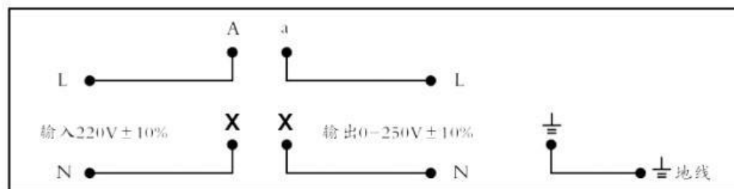
单相接线图
