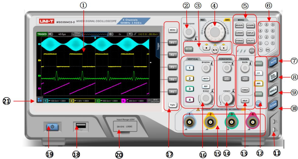
图 4-3 示波器前面板
