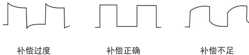
图 4-2 探头补偿校正
